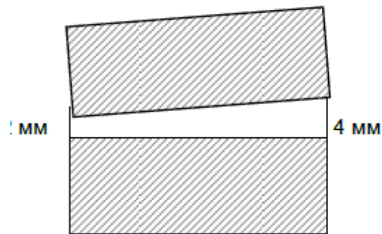
Вид спереди – горизонтальный монтаж
